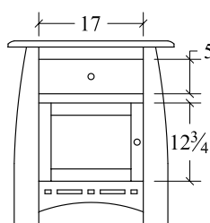
Nightstand (HYNSII) 1 drawer, 1 door 27w x 18d x 30h
