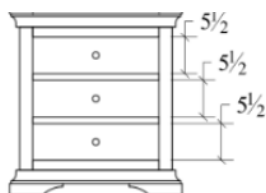
Nightstand (WTNS3) 3 drawer 26w x 16d x 28h
