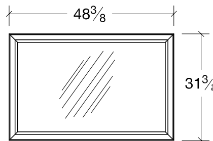
Mirror (ACMR48) 48½w x 31½h
